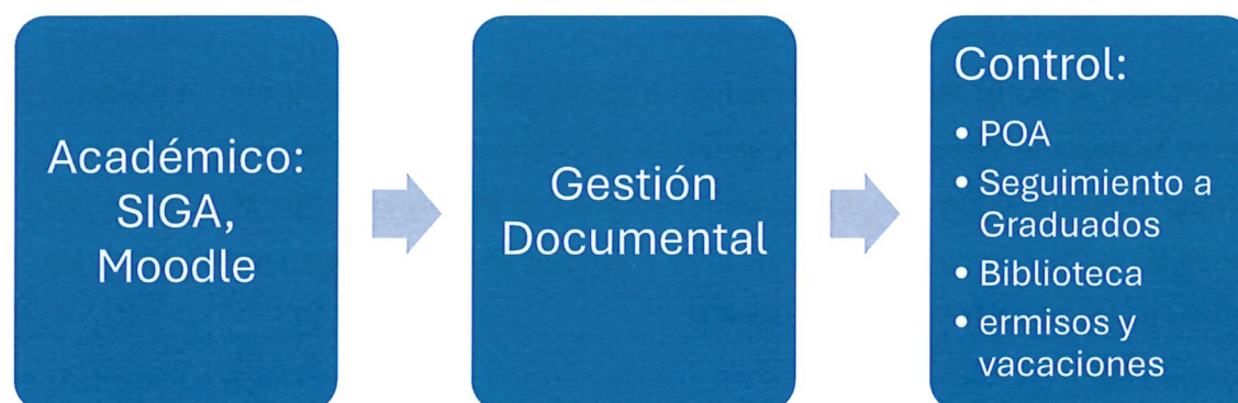
Ilustración 1. Herramientas SIG
